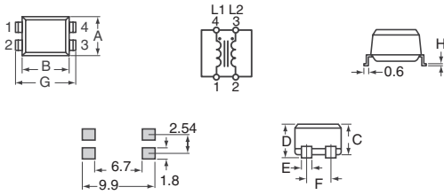
图 3 - ZJYS81R5-2PL25-G01、-2PL51-G01
