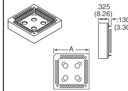
图 1 - 通孔安装
